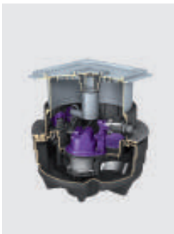
污水提升泵站 Aqualift F Compact
